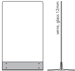
île 221 S w 750 x h 1250 x d 512mm w 29,52 x h 49,21 x d 20,15°
