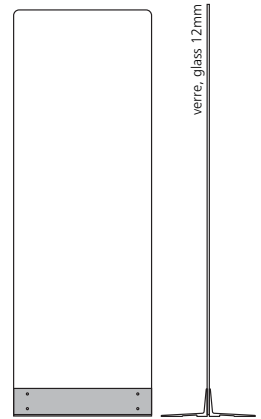
île 224 S w 750 x h 2200 x d 512mm w 29,52 x h 86,61 x d 20,15°
